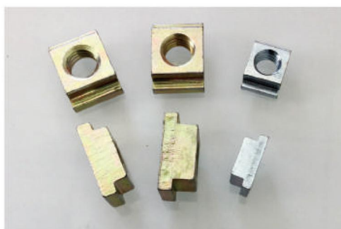
钣金螺母 Rivet Nut
